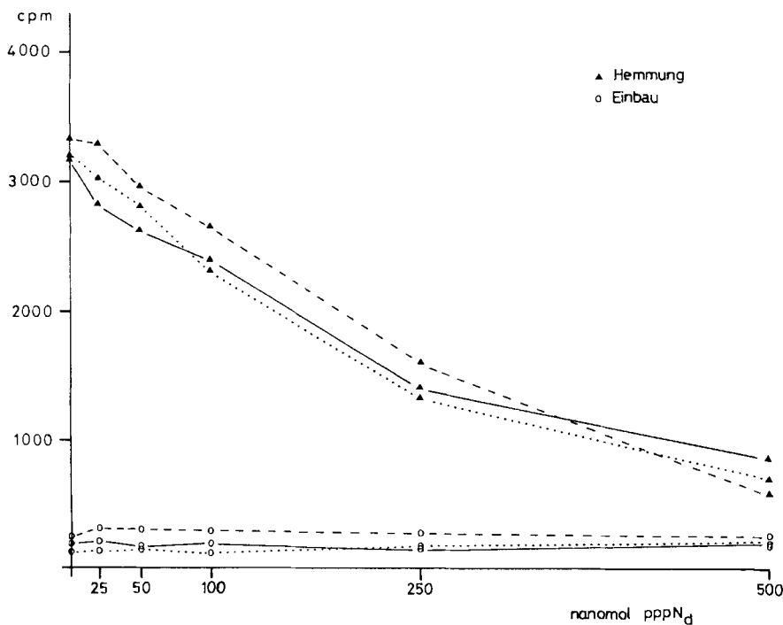
Fig. 2. Einbau- und Hemmungsversuche mit \text{pppN}_d (..... \text{pppM}_d , - - - - - \text{pppI}_d , ——— \text{pppZ}_d ) unter Verwendung von Poly[d(G-C)] als Matrice
