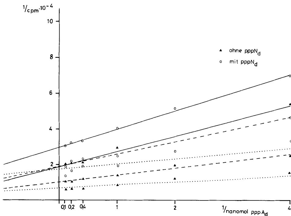
Fig. 3. Hemmwirkung des \text{pppN}_d ( . . . . . \text{pppM}_d , - - - - - \text{pppI}_d , ——— \text{pppZ}_d ) in Abhängigkeit von \text{pppC}_d nach Lineweaver-Burke
